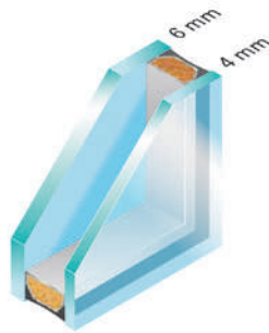
Schallschutzglas 36 dB Ug-Wert = 1,1 W/m²K
