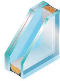
Sicherheitsglas (P2A) Ug-Wert = 1,1 W/m²K
