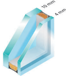
Schallschutzglas 39 dB Ug-Wert = 1,1 W/m²K
