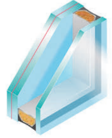
Sicherheitsglas (P4A) Ug-Wert = 1,1 W/m²K
