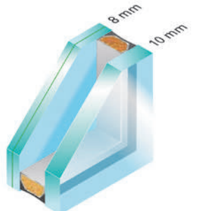
Schallschutzglas 45 dB Ug-Wert = 1,1 W/m²K
